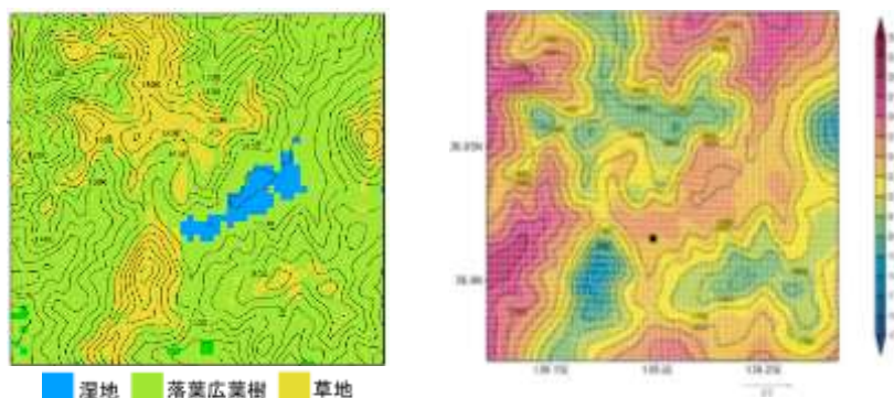
図 1 Case2 における土地利用入力図（左図）と 8 月 3 日 15 時の気温分布（右図）
